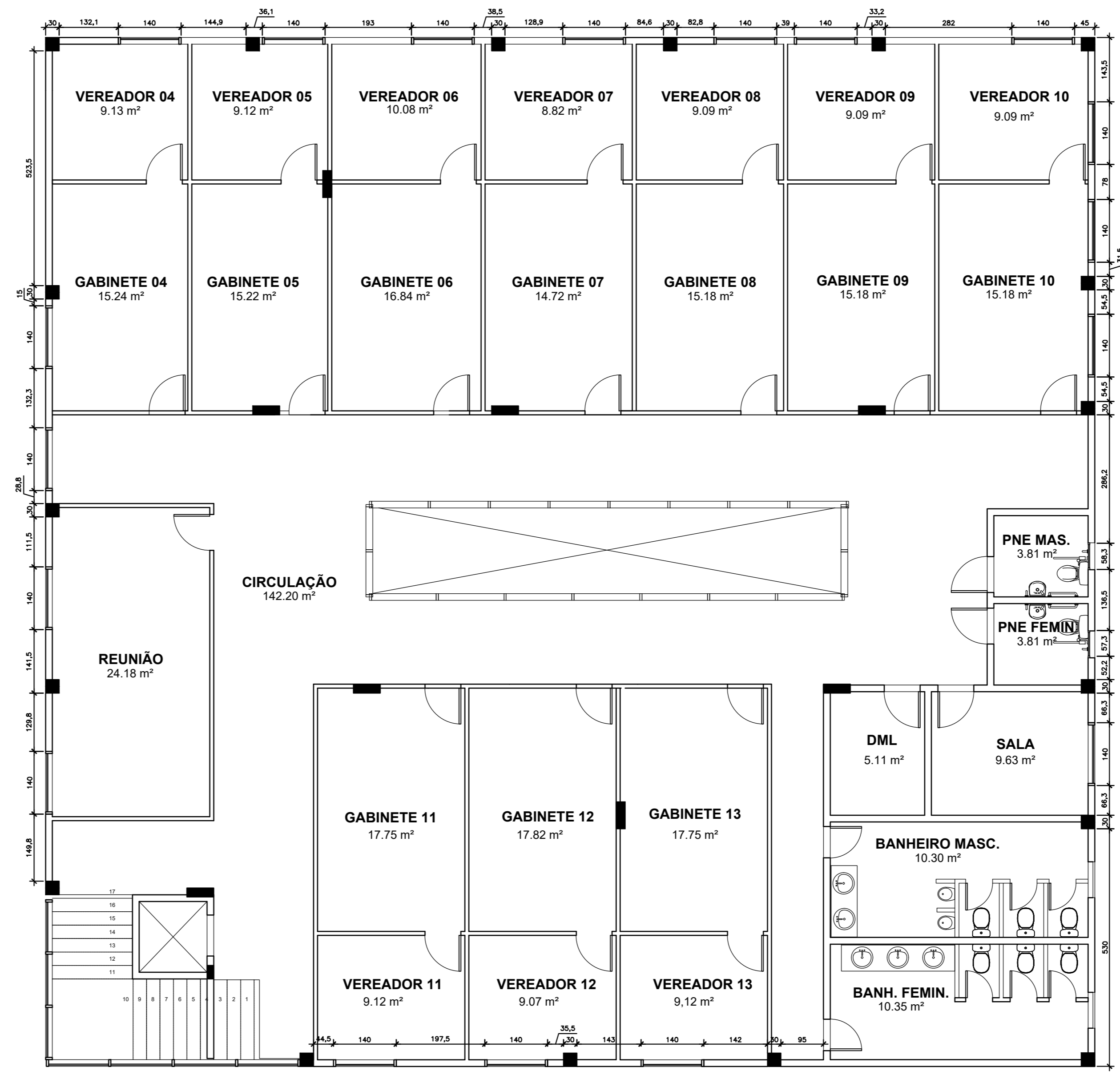
PLANTA BAIXA 2º PAVIMENTO ESCALA 1/75
