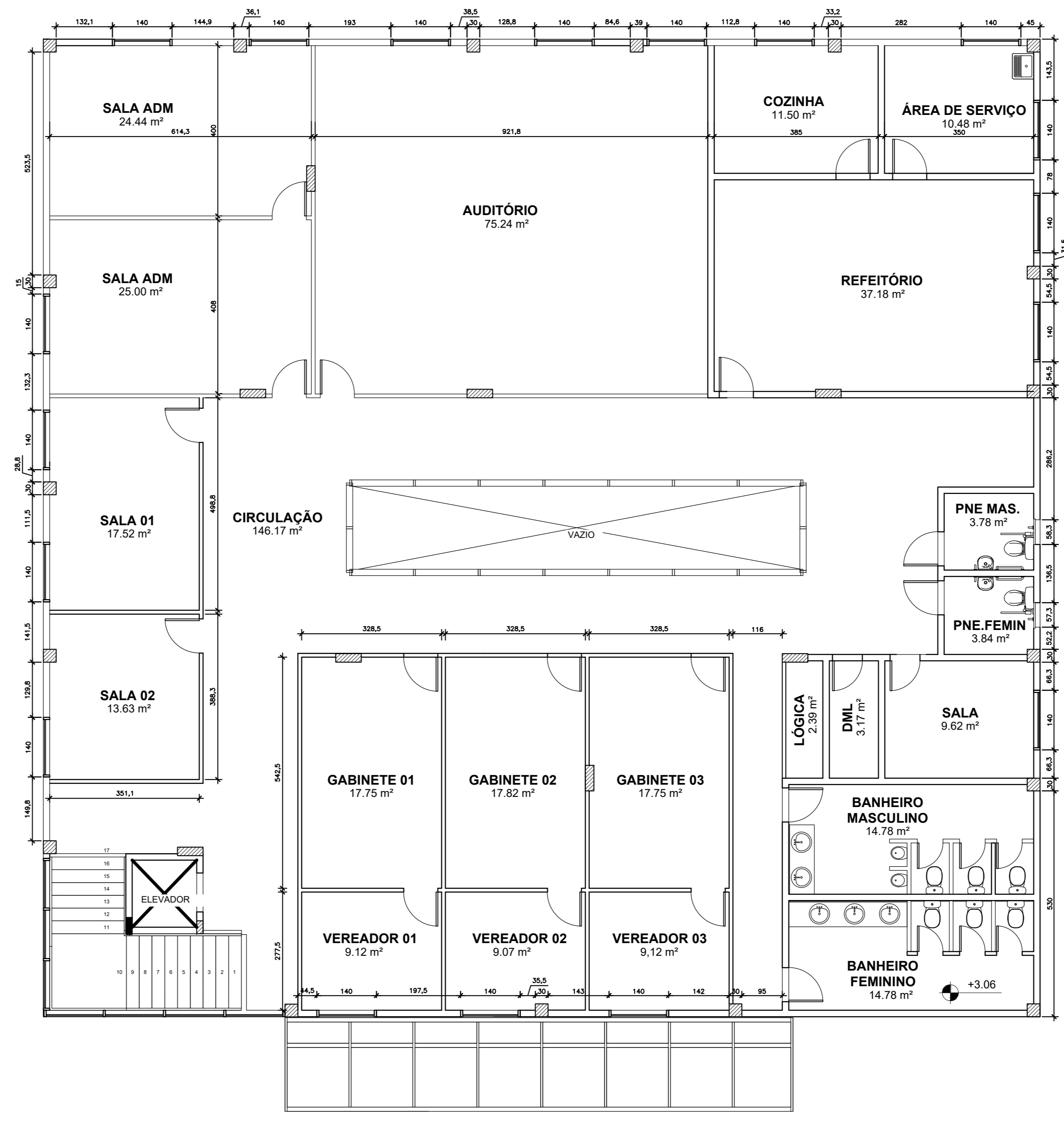
PLANTA BAIXA 1º PAVIMENTO ESCALA 1/75
